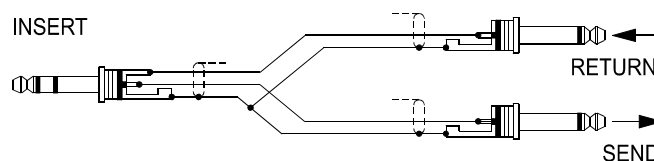
Abbildung 2-3: Y-Kabel für die Verwendung der Insert-Buchse
