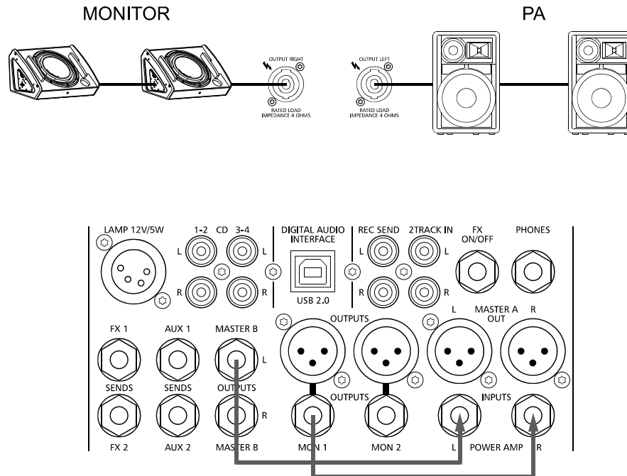
Abbildung 6-4: Mono PA + Monitor
