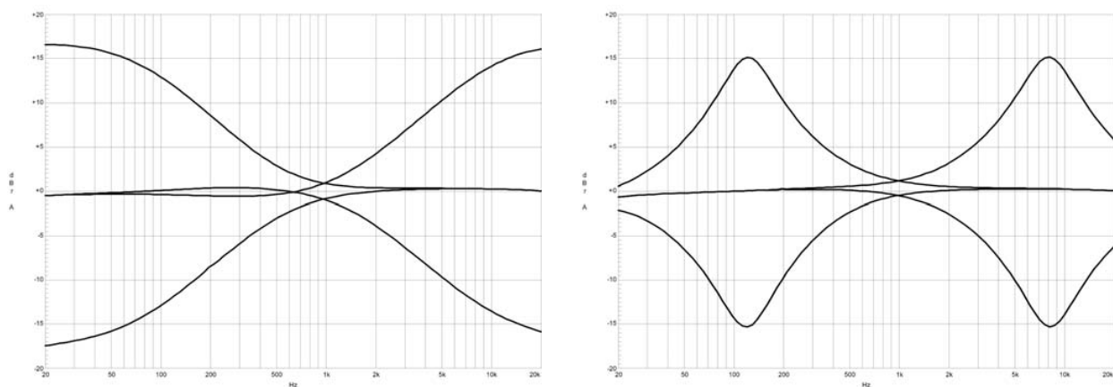
Abbildung 2-7: Frequenzgang des LO/HI-Filters bzw. des MID-Filters
