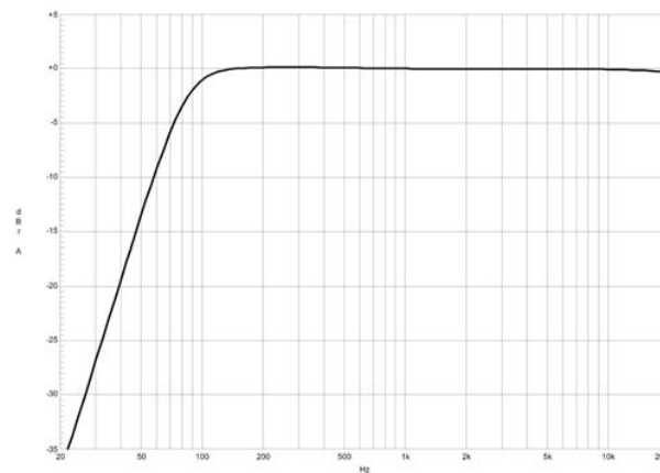
Abbildung 2-5: Frequenzgang des LO CUT Filters
