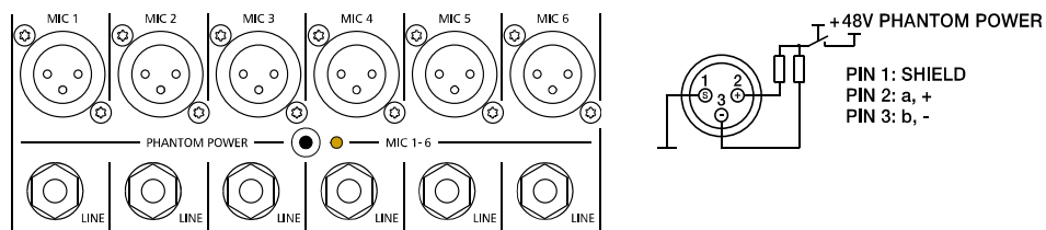
Abbildung 2-1: Mikrofon-Eingänge
