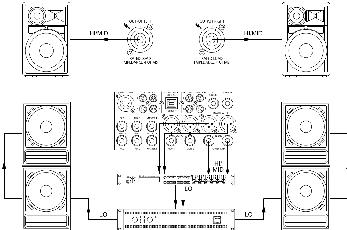
Abbildung 6-5: Aktiv Stereo 2-Weg System
