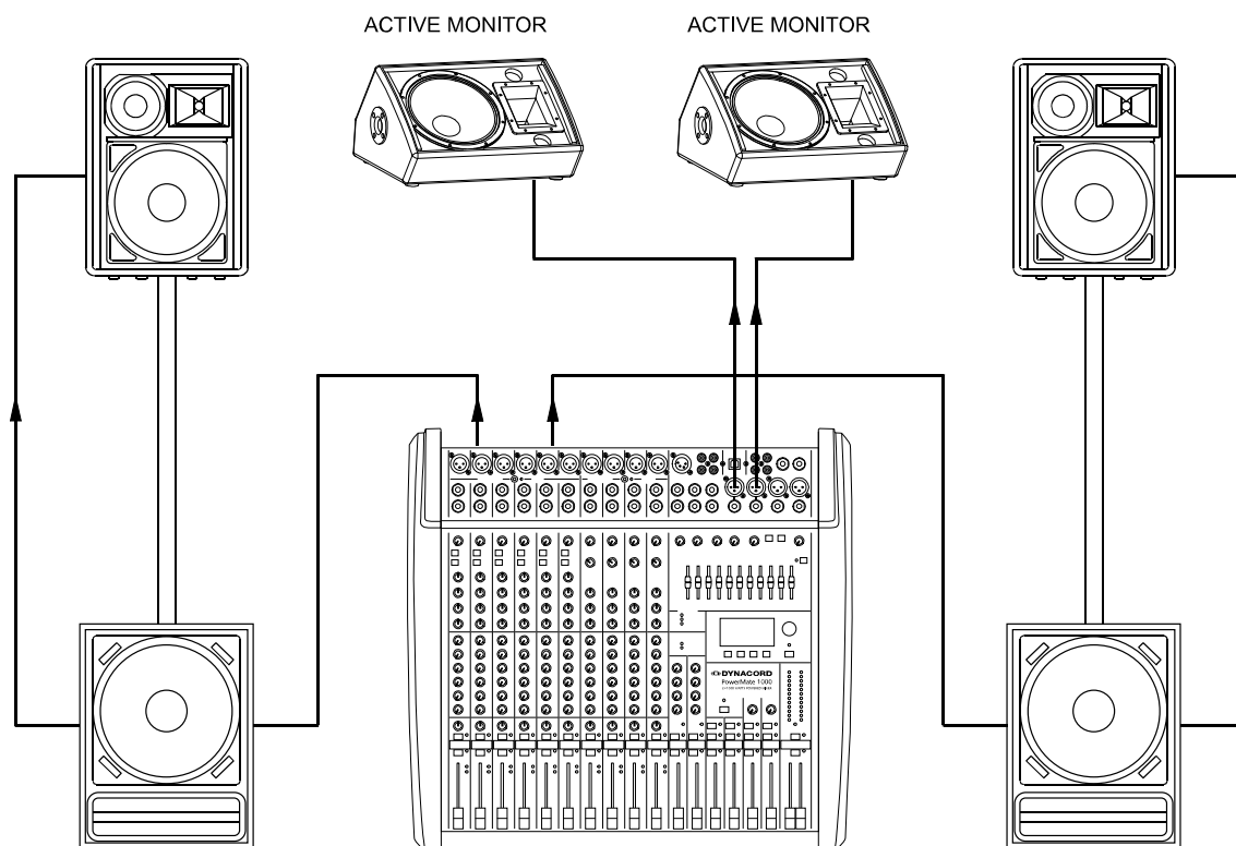
Abbildung 5-1: Aufbau einer Standard-PA
