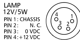
Abbildung 2-17: Belegung der LAMP 12V/5W-Buchse
