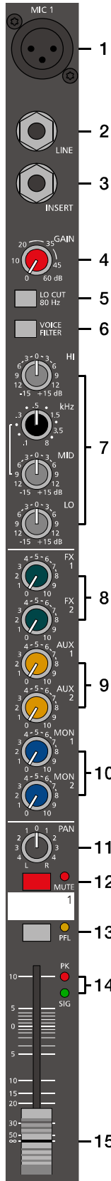
Abbildung 2-1: Mikrofon-Eingänge
