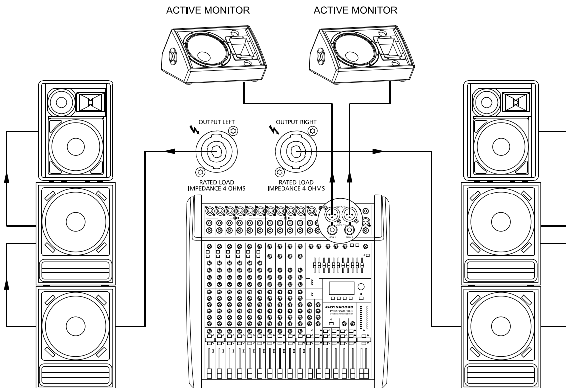
Abbildung 6-1: Maximale Ausbaustufe, Passivbetrieb
