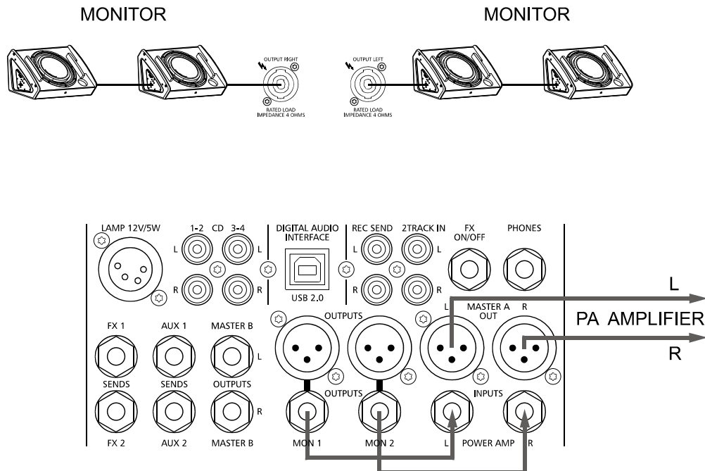
Abbildung 6-3: Verwendung der internen Endstufen für Monitore
