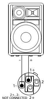
Abbildung 2-19: Anschlussbeispiel einer passiven Lautsprecherbox
