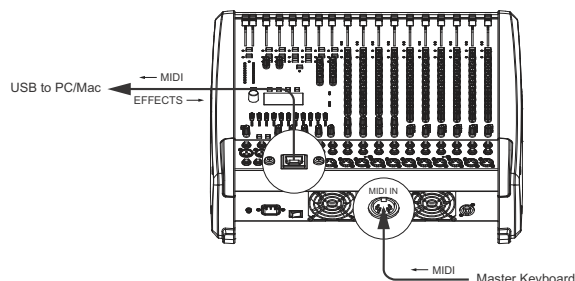
Abbildung 4-10: PC/Mac als MIDI-Klangerzeuger
