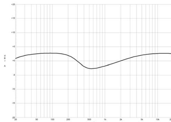
Abbildung 2-6: Frequenzgang des Voice-Filters
