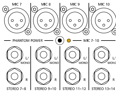
Abbildung 2-8: Mikrofon-Eingänge (Stereo)
