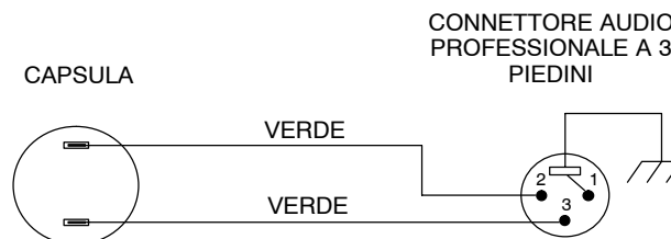
CONNESSIONI INTERNE
