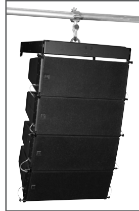
Abb. 17: Hochfahren der oberen vier CAD 208-Boxen
