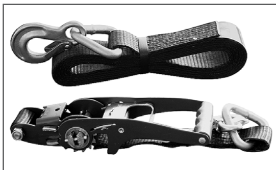
Abb. 10: Zurrkord zum Curven des Arrays im Compression Mode
